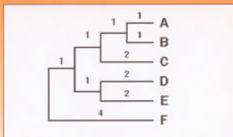
Figura 3 - Similarità genetica tra singoli soggetti utilizzando le analisi del DNA
